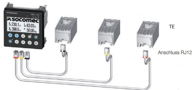
DIRIS A-40
