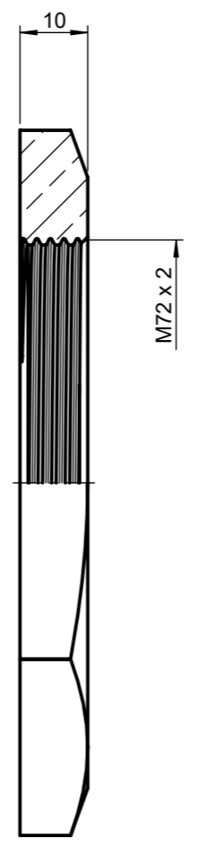
A-A (1 : 1)
